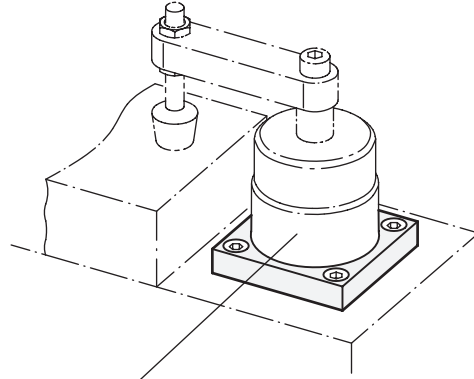
GN 876 Döner kelepçeler
